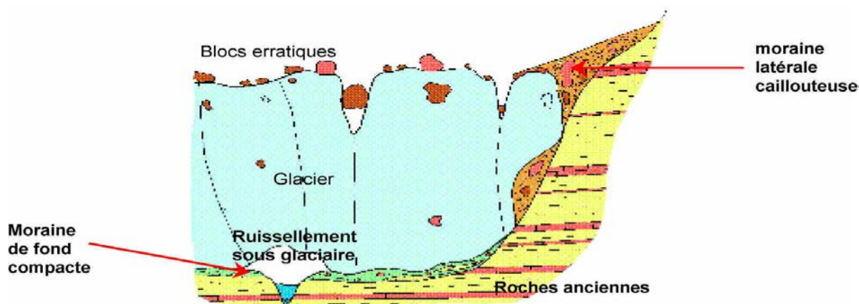
Figure 9 : Coupe schématique d'un glacier
