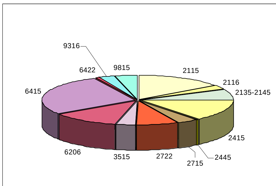
Figure 13 : Diagramme de répartition des surfaces des sols sur le secteur
