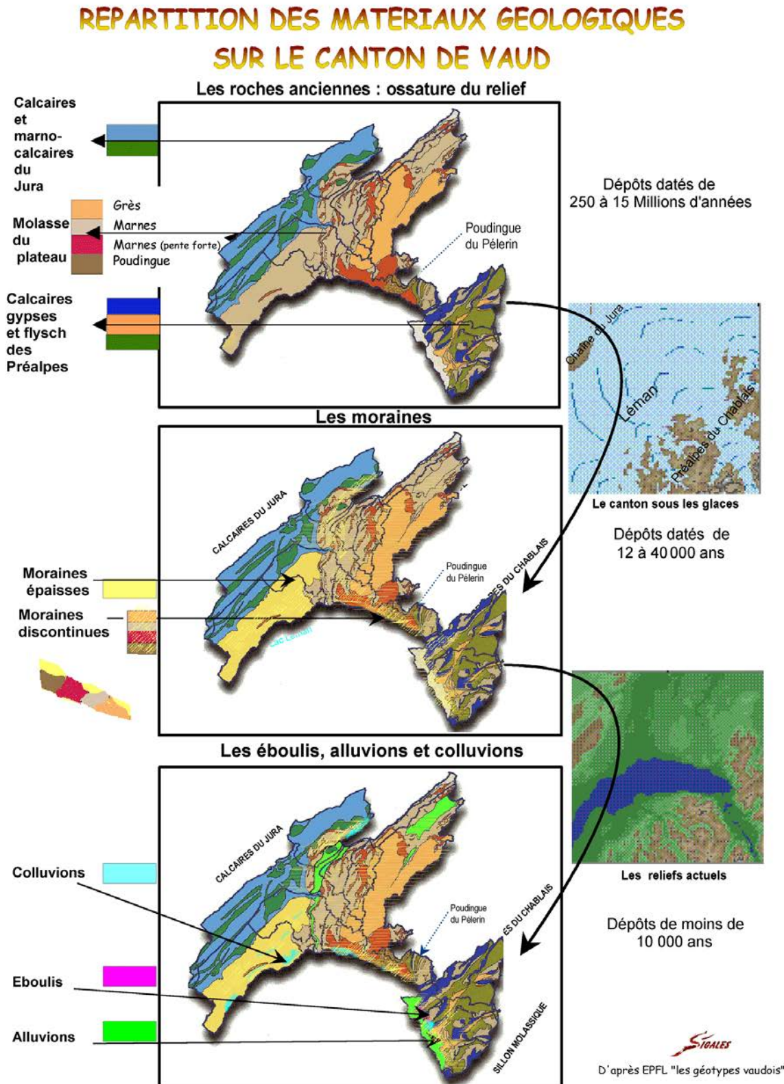
Figure 1 : Schéma de la mise en place des différentes roches mères du canton de Vaud
