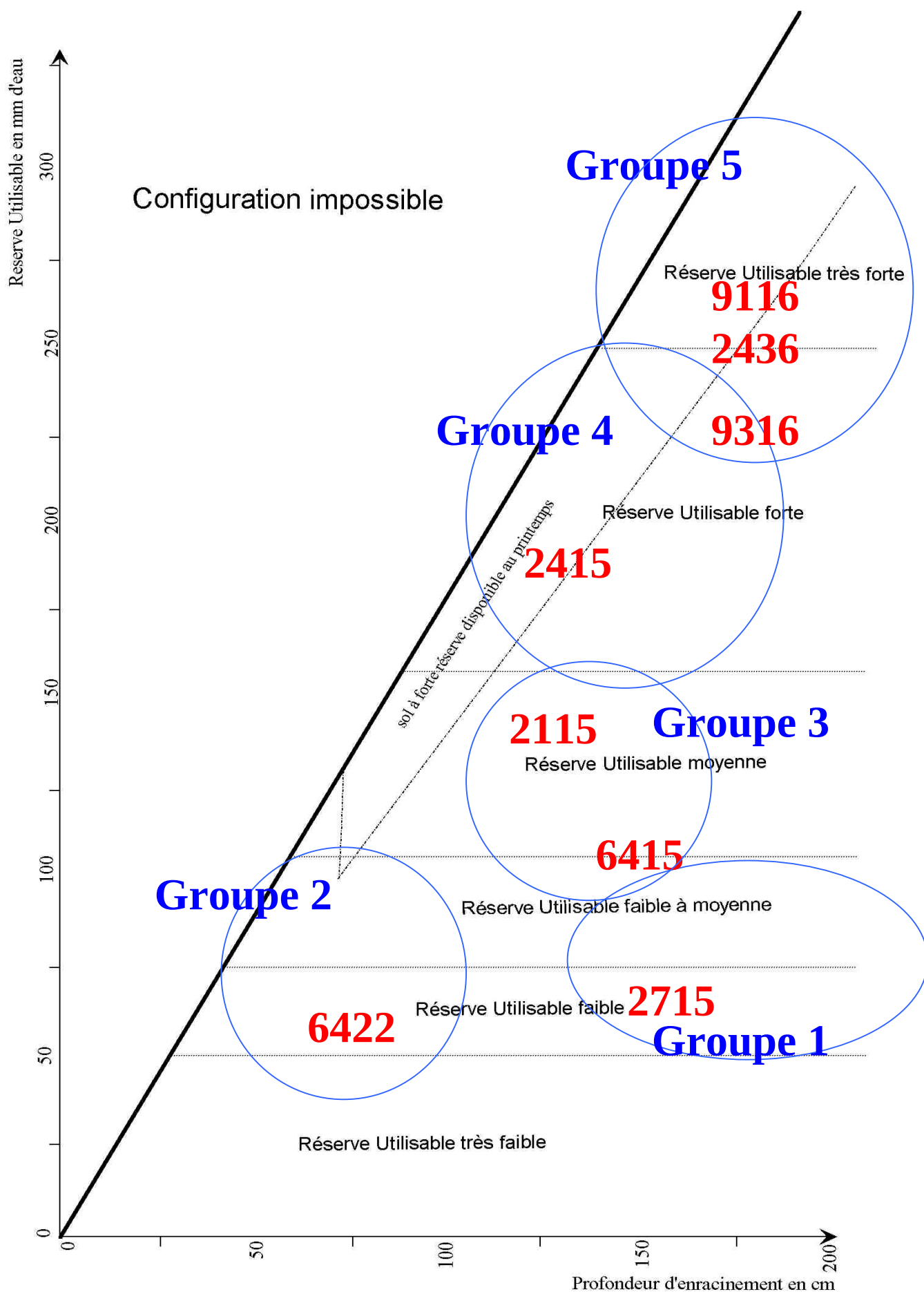
Figure 14 : Répartition des sols en fonction de leur réserve utilisable et de leur profondeur d'enracinement
